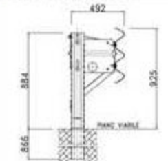
Barriera H2BL500-arg.
