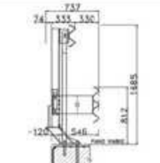
Barriera H3BP100
